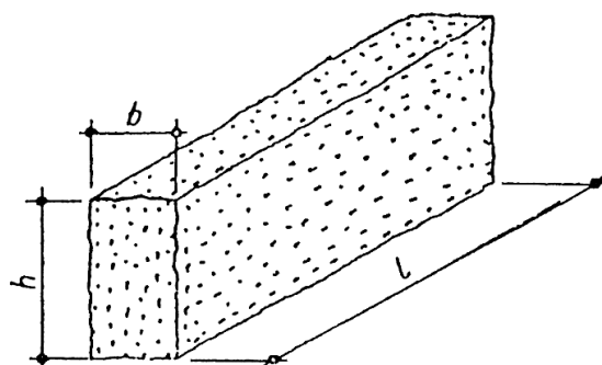
Krawężnik drogowy rodzaju A
